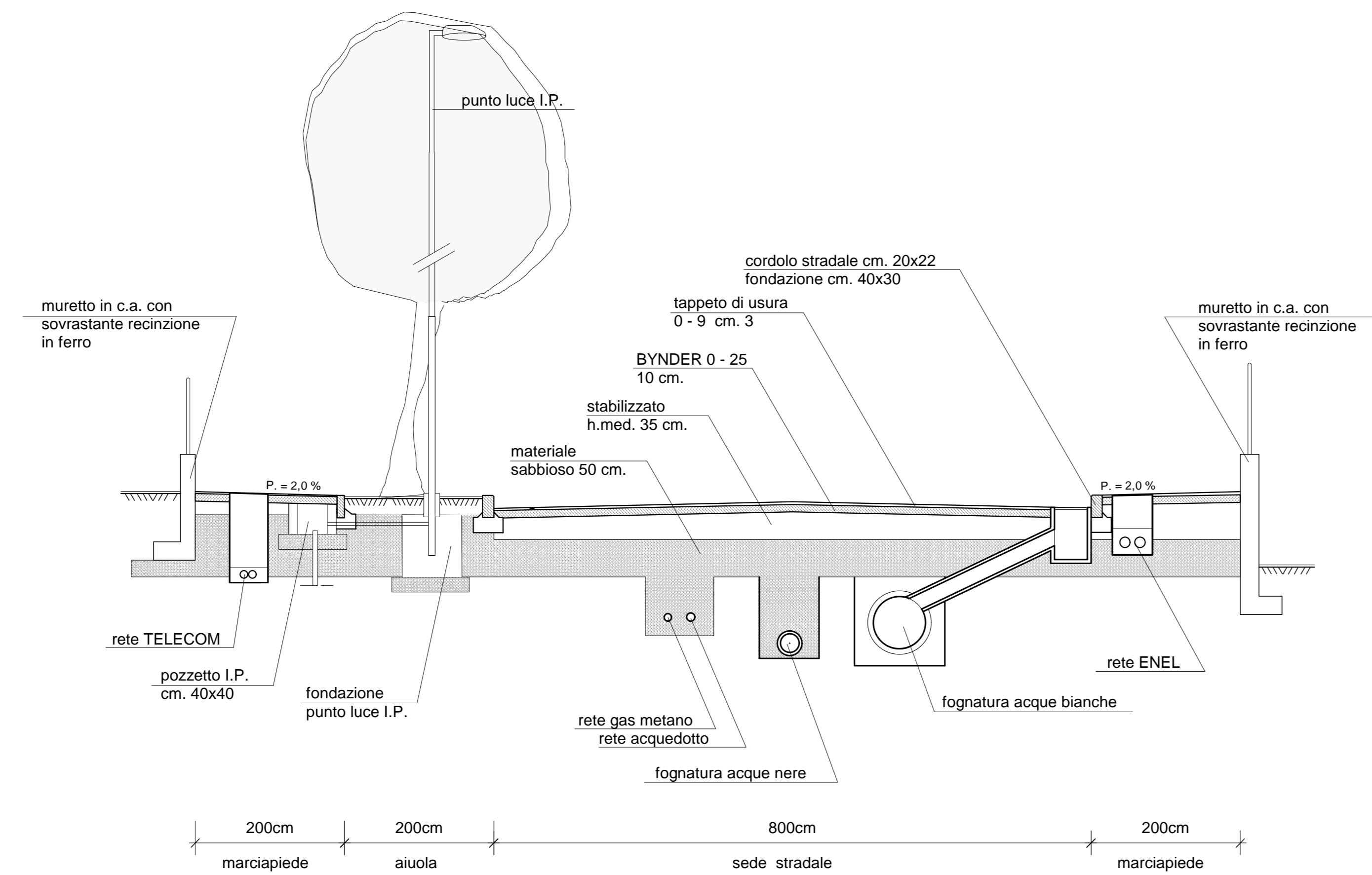
Sezione TIPO 1 Scala 1:50
