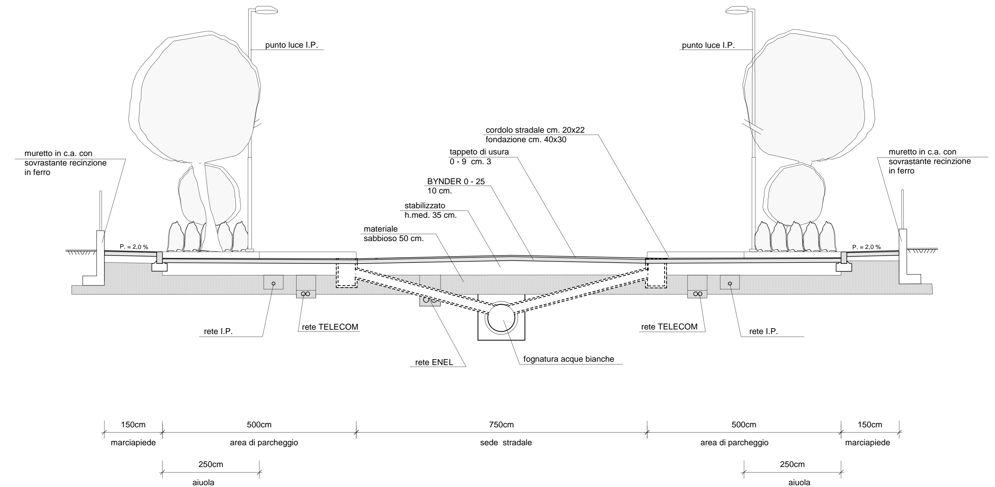
Sezione TIPO 2 Scala 1:50
