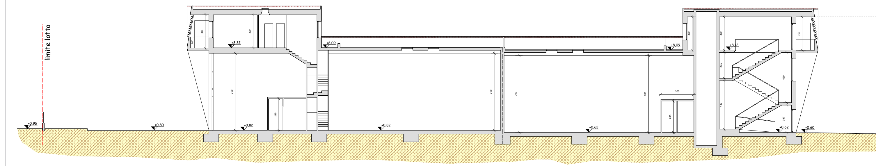
SEZIONE A - A
