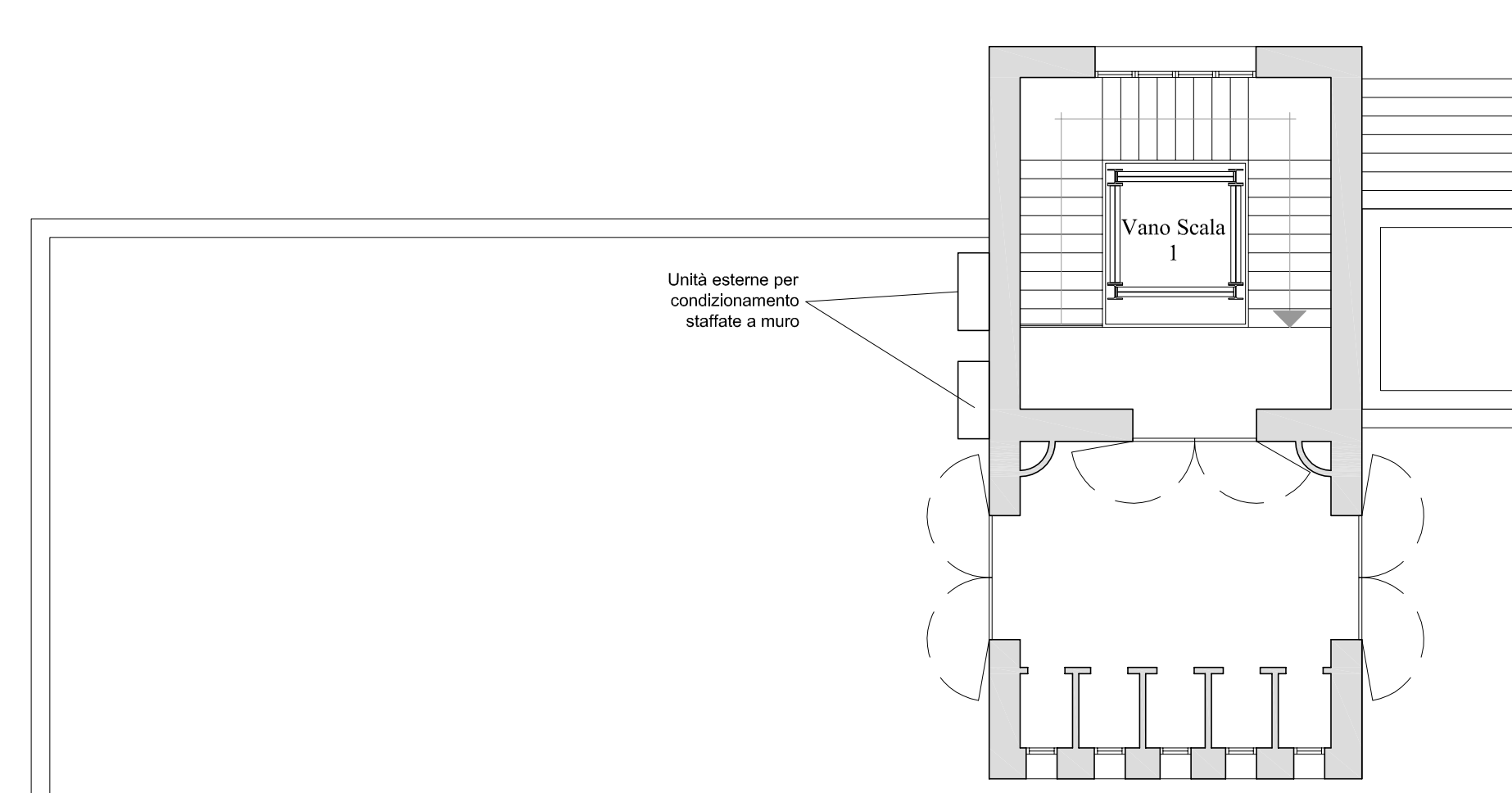
MACCHINE ESTERNE CONDIZIONAMENTO scala 1:100
