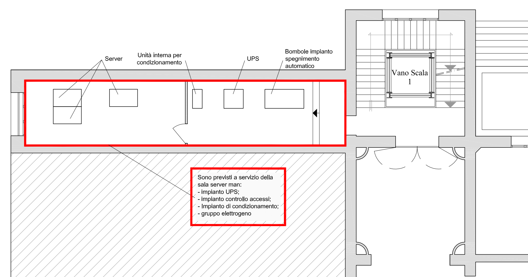
IMPIANTI SPECIALI SALA SERVER MAN scala 1:100
