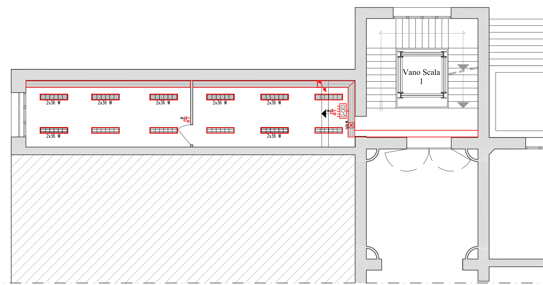
IMPIANTO ELETTRICO SALA SERVER MAN scala 1:100
